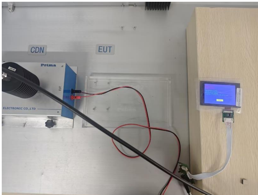
图 6-5 传导抗扰度测试图
