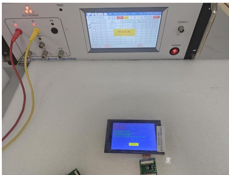
图 6-4 脉冲群测试图
