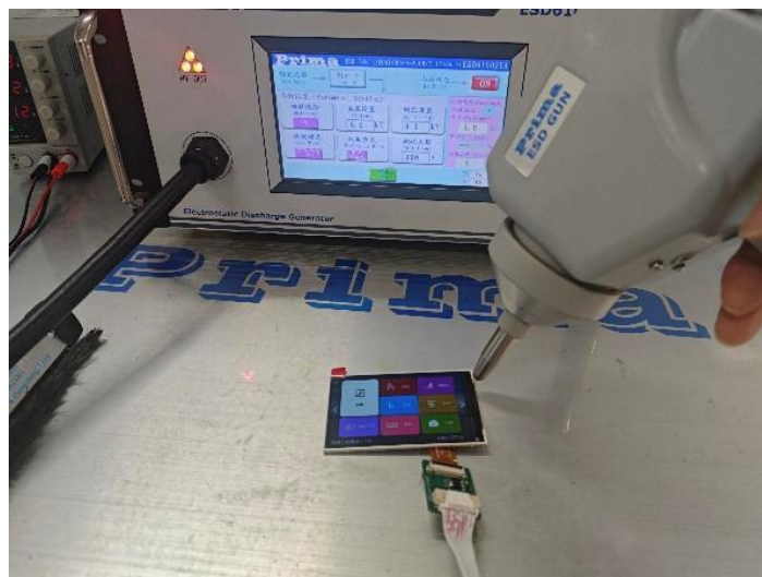
图 6-2 ESD 测试图
