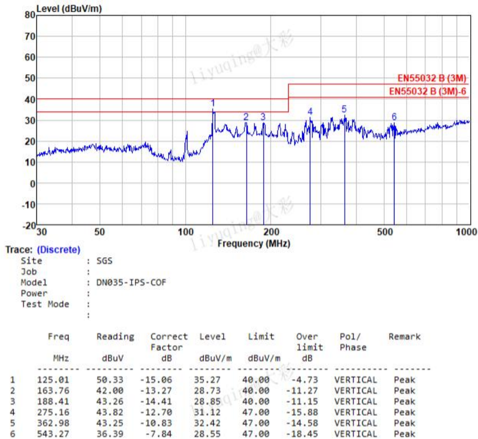
图 6-8 辐射测试垂直方向
