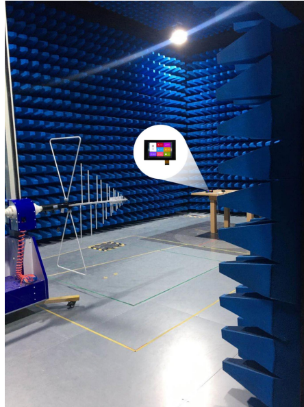
图 6-6 辐射测试图
