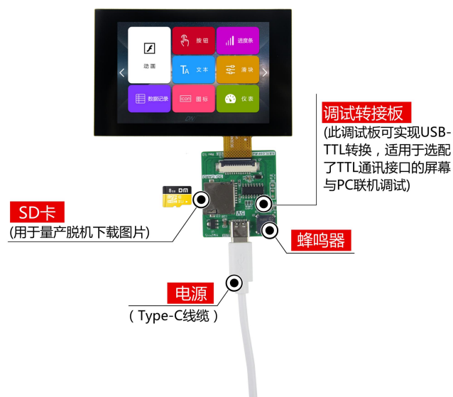
图 1-4 调试工具图
