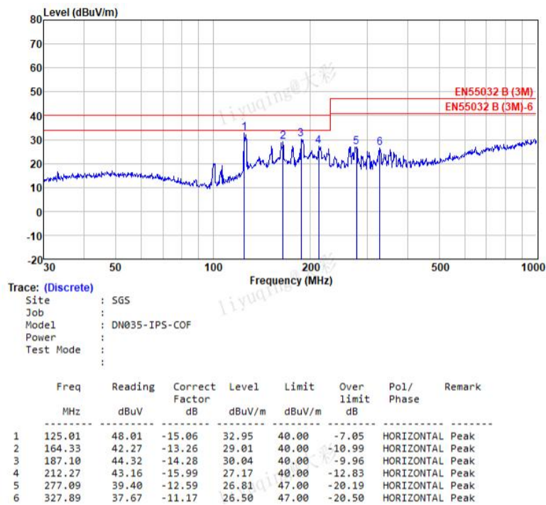
图 6-7 辐射测试水平方向
